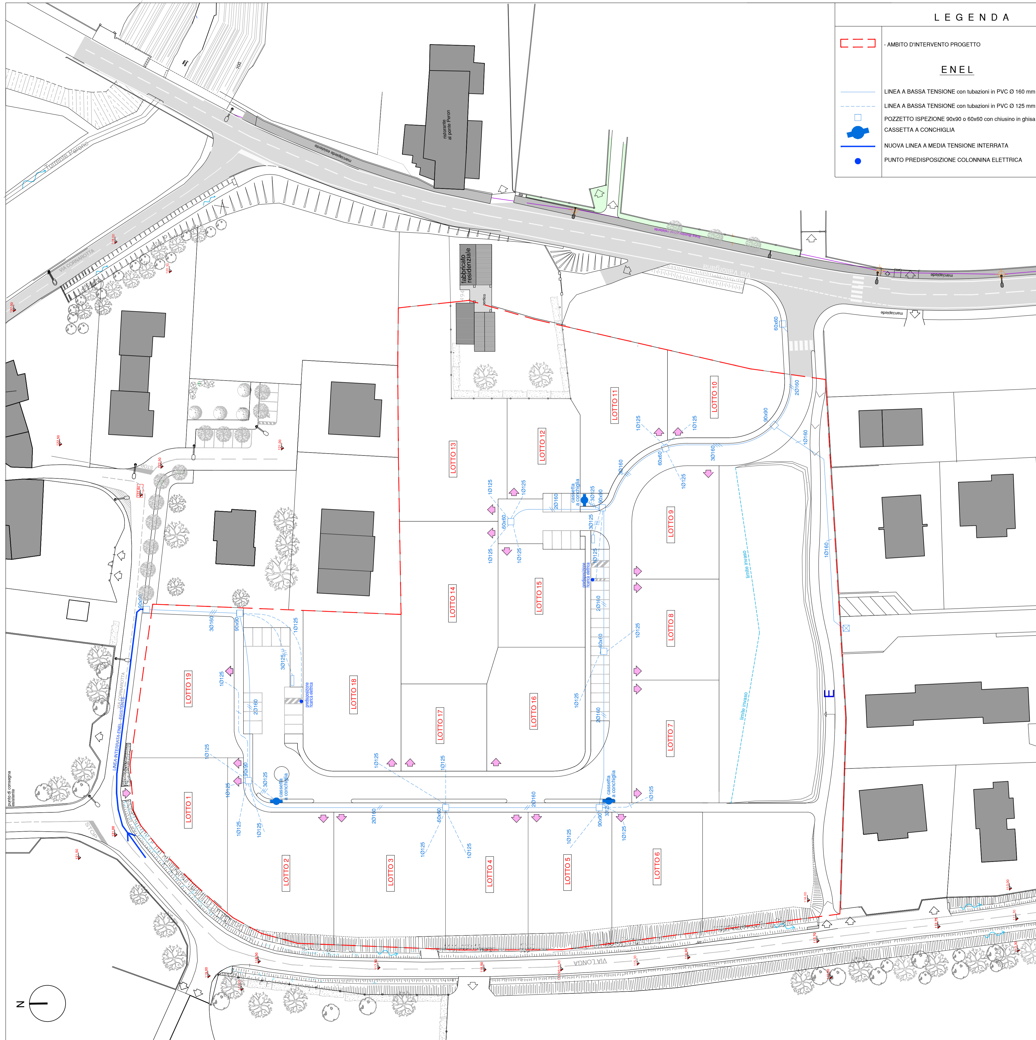
PLANIMETRIA DELLO STATO DI PROGETTO - 1:500
